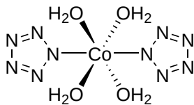
图 7: \text{Co}(\text{N}_5)_2(\text{H}_2\text{O})_4 的结构
